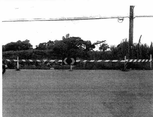
FOTO 04 - Implantação de sinalização com cavaletes no desbarrancamento
