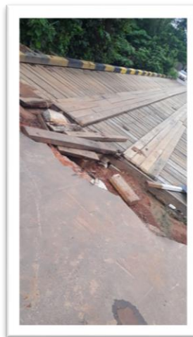
Figura 2 – Reparos na cabeceira da ponte.
